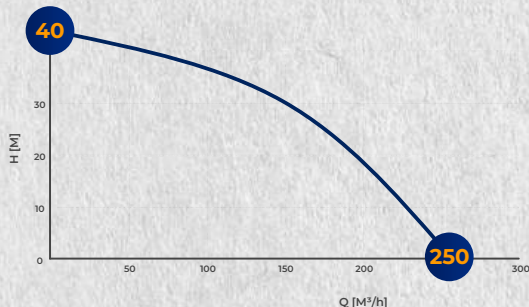
SE HC / 100 | CURVA DE APLICAÇÃO
